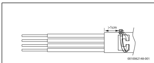
Fig. 34 Fixation du serre-câble sur le câble
