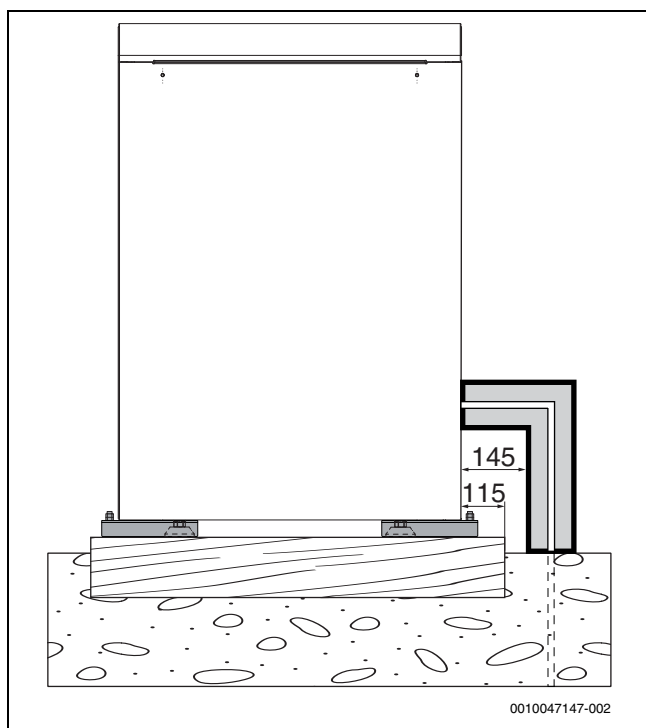
Fig. 21 Vue latérale avec kit d'installation
