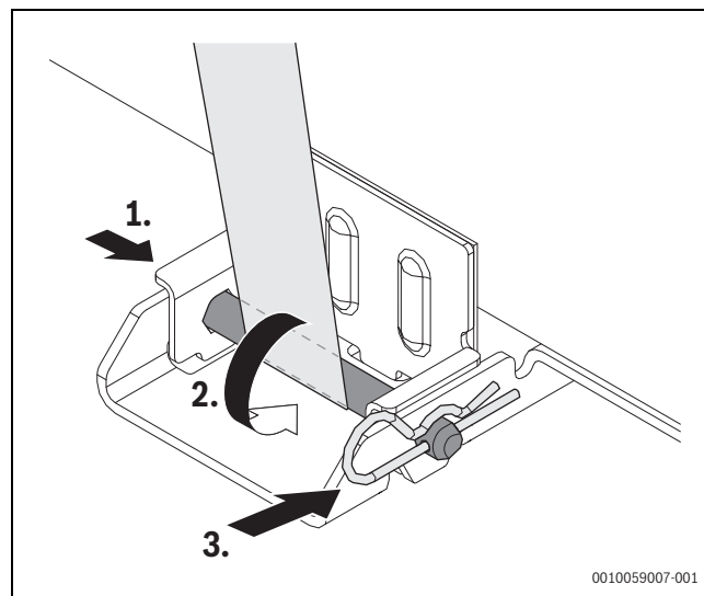
Fig. 10 Insertion du support de verrouillage, de la broche et de la sangle
