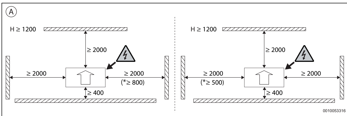
Fig. 16 Écarts à respecter pour l'installation
