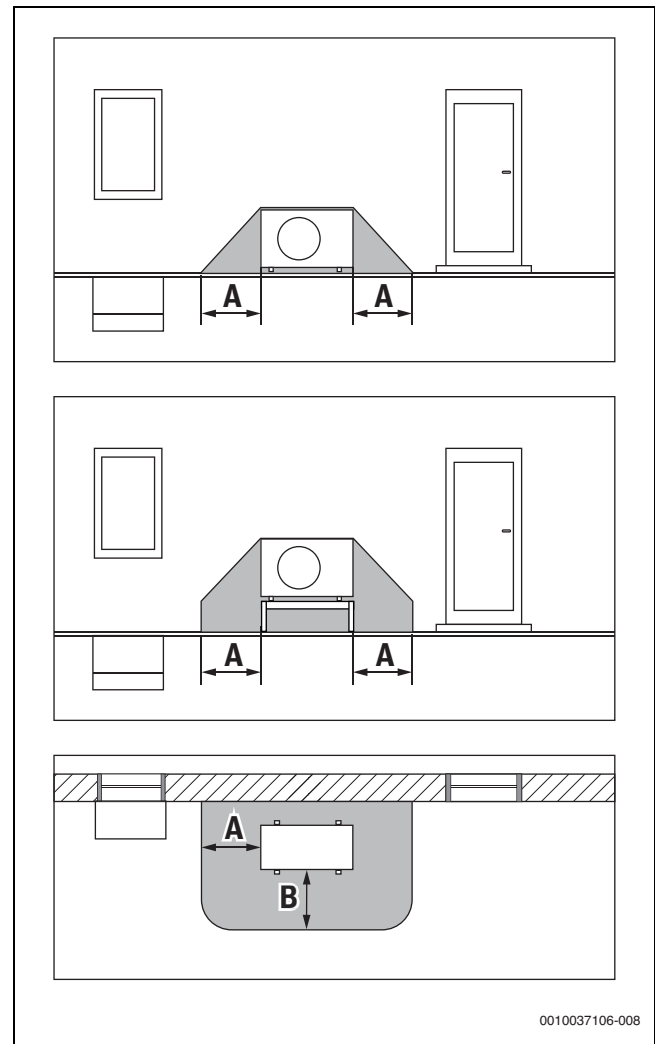
Fig. 7 Zone de protection placée au sol
