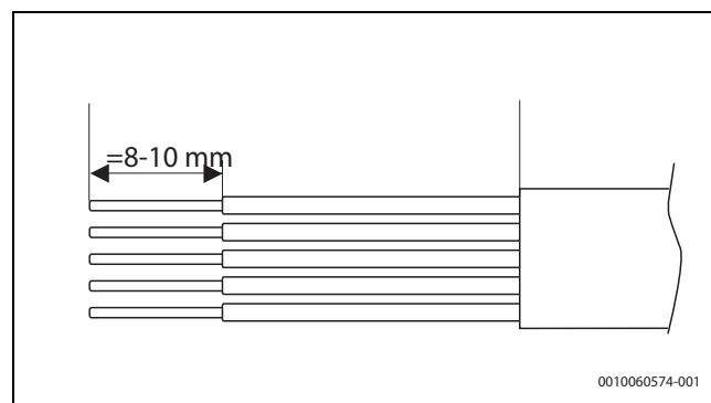
Fig. 32 Alimentation électrique : longueur de dénudage du fil
