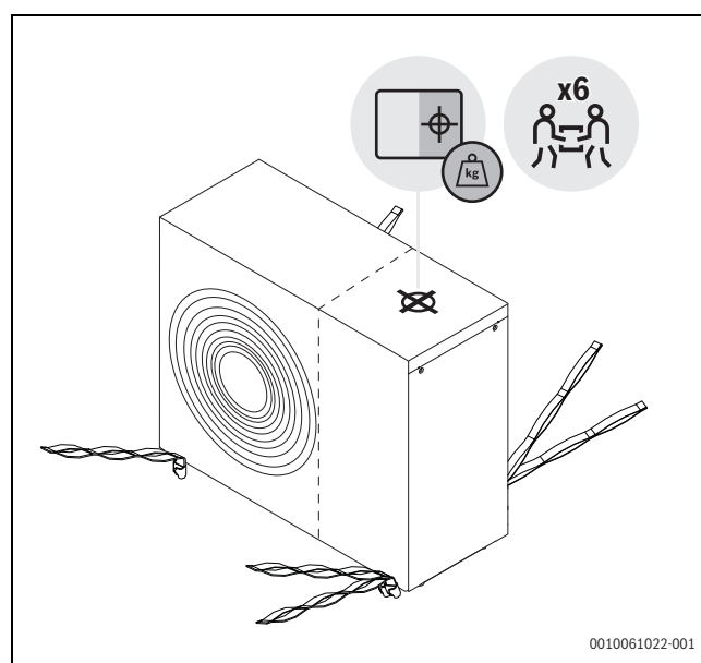
Fig. 11 Utilisation des sangles fournies pour transporter la pompe à chaleur sans son emballage
