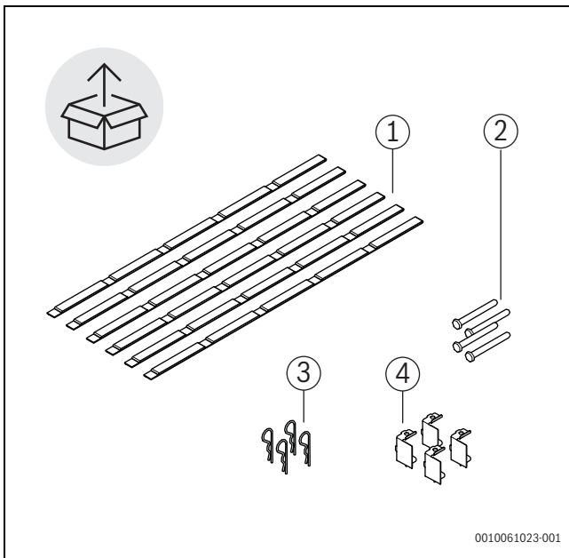
Fig. 12 Pièces pour le transport de l'appareil
