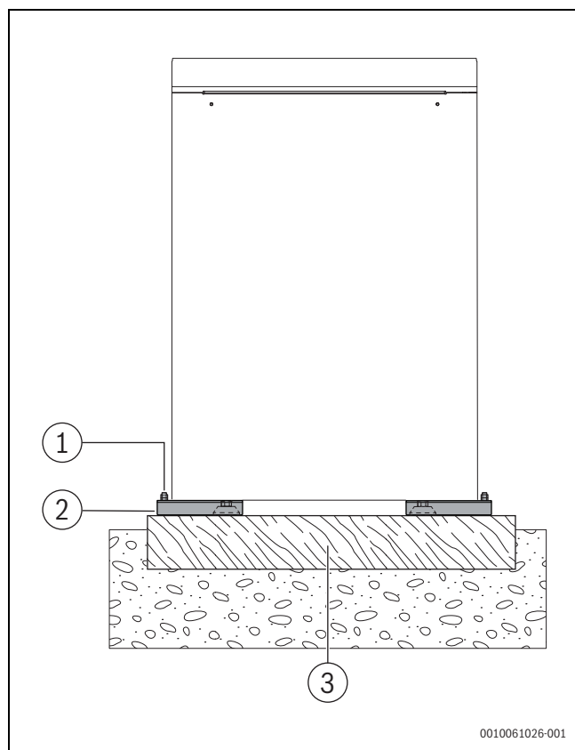
Fig. 18 Fixation de la pompe à chaleur
