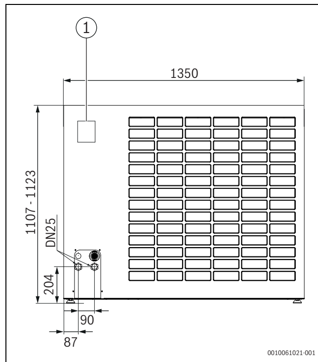
Fig. 4 Dimensions et raccords de la pompe à chaleur, arrière
