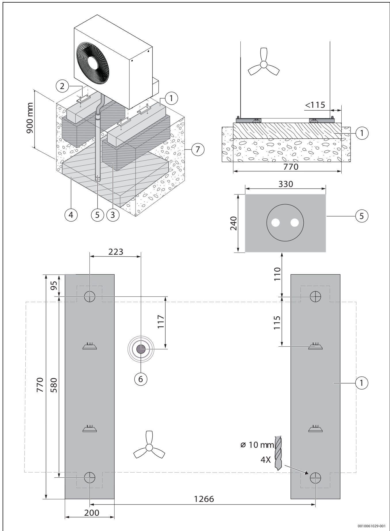
Fig. 22 Plan de fondation, situation 1
