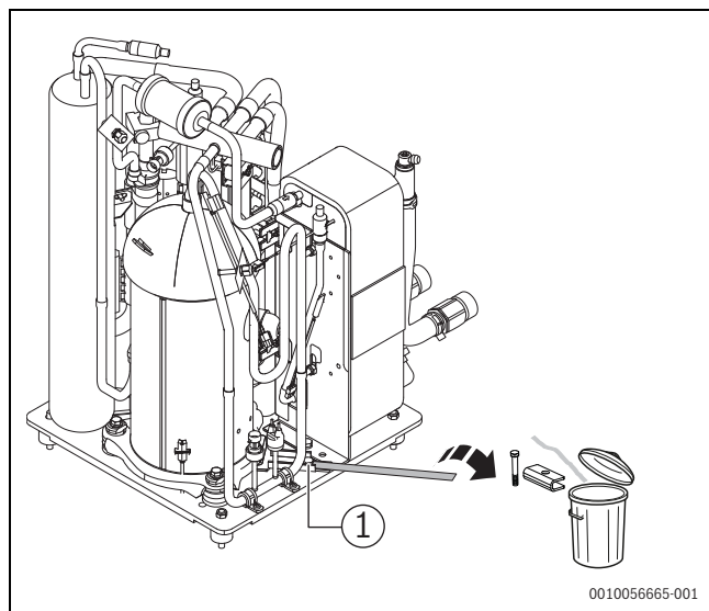
Fig. 29 Sécurisations pour le transport
