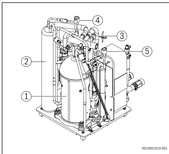
Fig. 2 Vue d'ensemble du produit - vue avant
