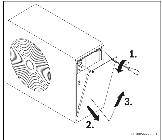
Fig. 27 Couvercle latéral
