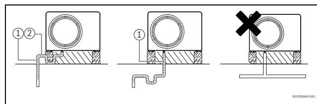
Fig. 25 Écoulement des condensats vers les égouts ou l'évacuation des eaux pluviales
