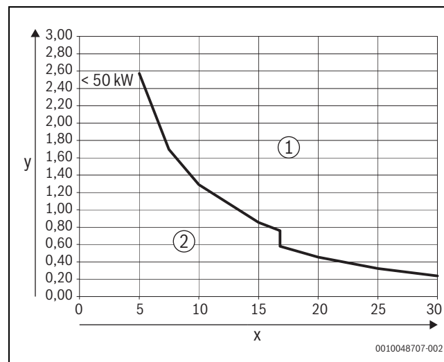
Fig. 17 Générateurs de chaleur < 50 kW – 100 kW
