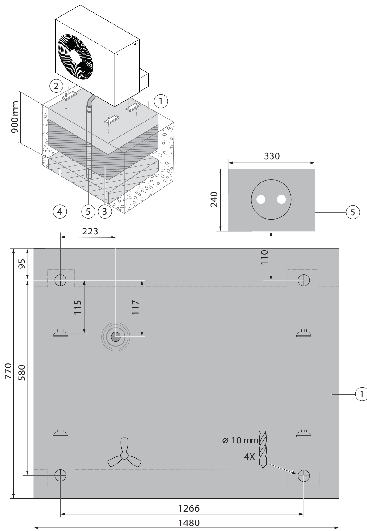
Fig. 23 Plan de fondation, situation 2
