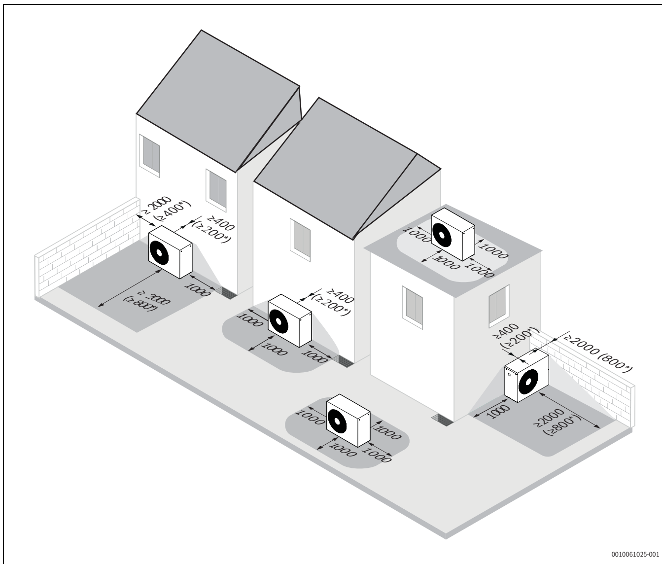
Fig. 15 Espacement recommandé entre la pompe à chaleur et les objets fixes voisins (mm)
