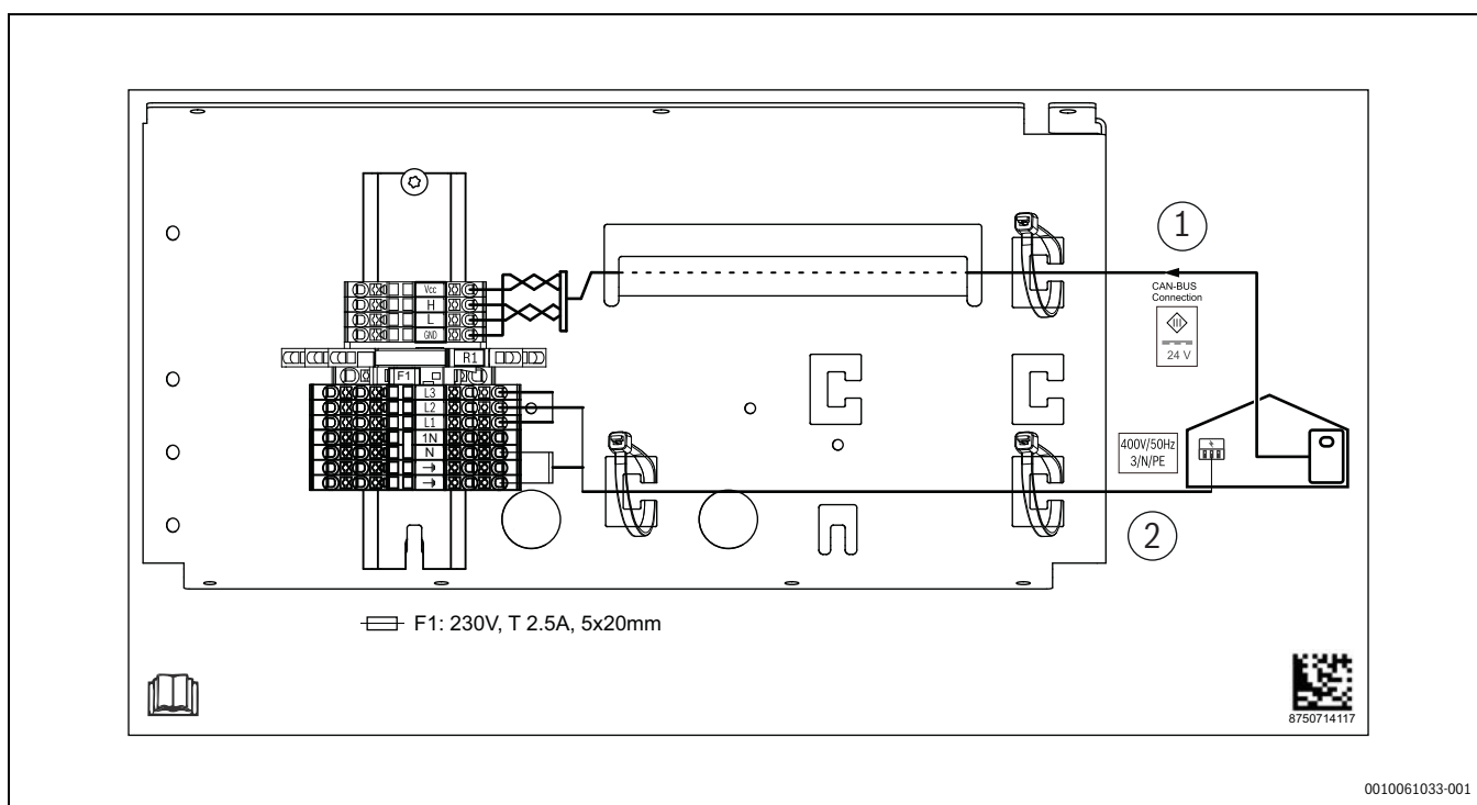
Fig. 33 Bornes de raccordement dans la zone de raccordement de l'installation
