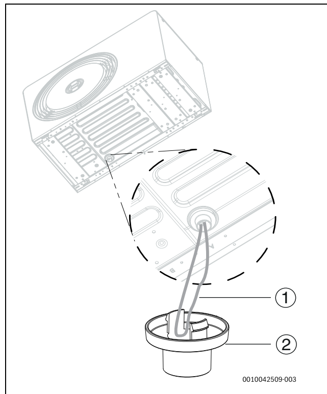
Fig. 24 Installation du raccord d'évacuation
