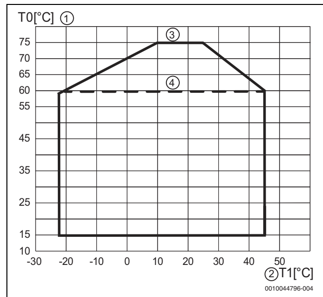
Fig. 4 Pompe à chaleur en mode chauffage sans chauffage auxiliaire
