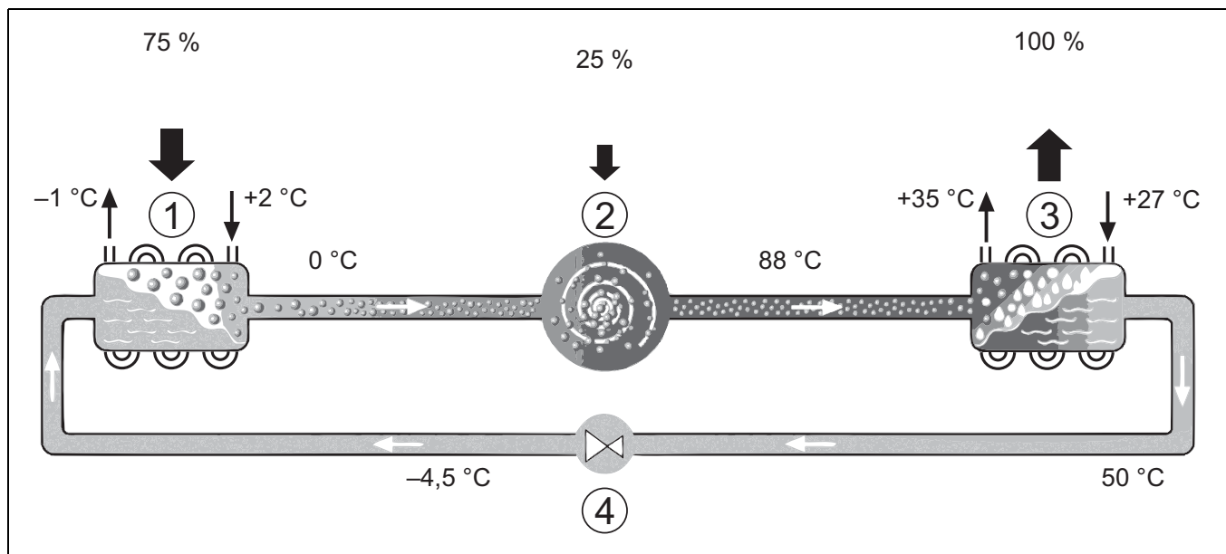
Fig. 5 Principe fonctionnel du circuit de réfrigérant dans la pompe à chaleur
