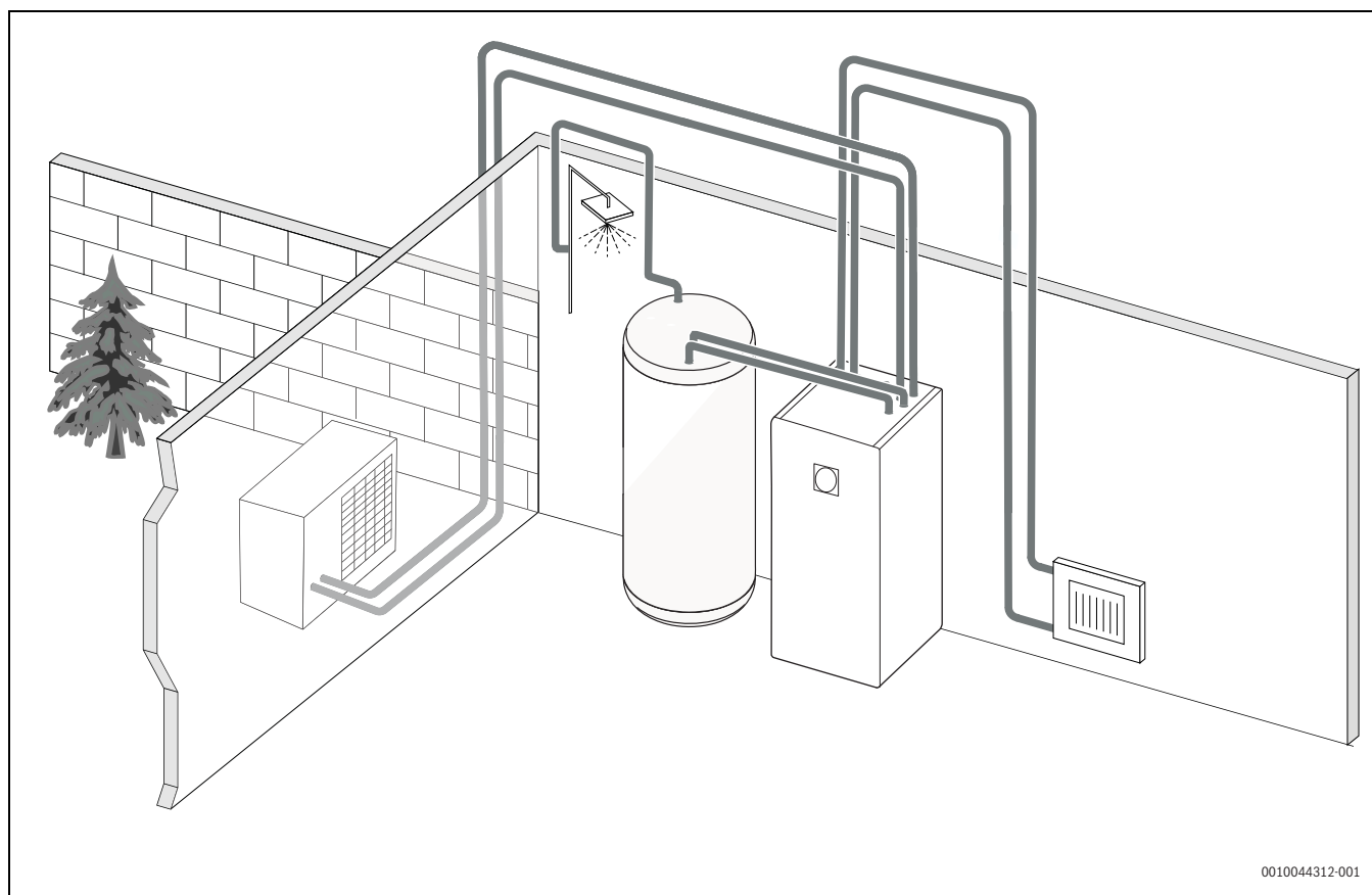
Fig. 7 Unité extérieure AW OR, unité intérieure Compress 5800iAW/6800iAW 12 MB avec ballon tampon intégré
