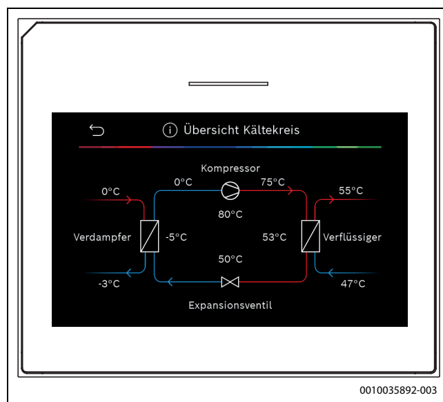
Bild 10 Übersicht Kältekreis
