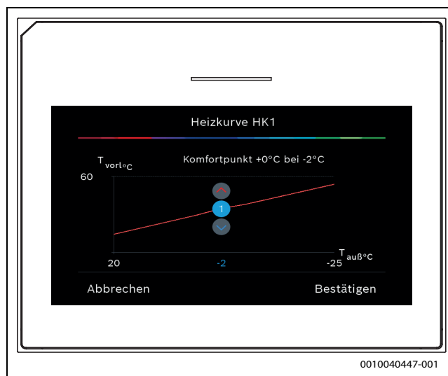
Bild 4 Komfortpunkt (nur wenn die Regelungsart auf Außentemperatur mit Fußpunkt eingestellt ist) für Einstellung mit zusätzlichem Fußpunkt einstellen
