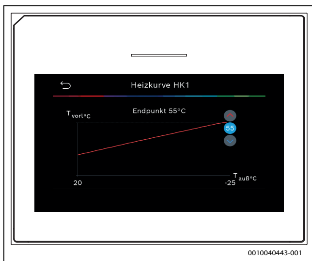
Bild 5 Endpunkt einstellen
