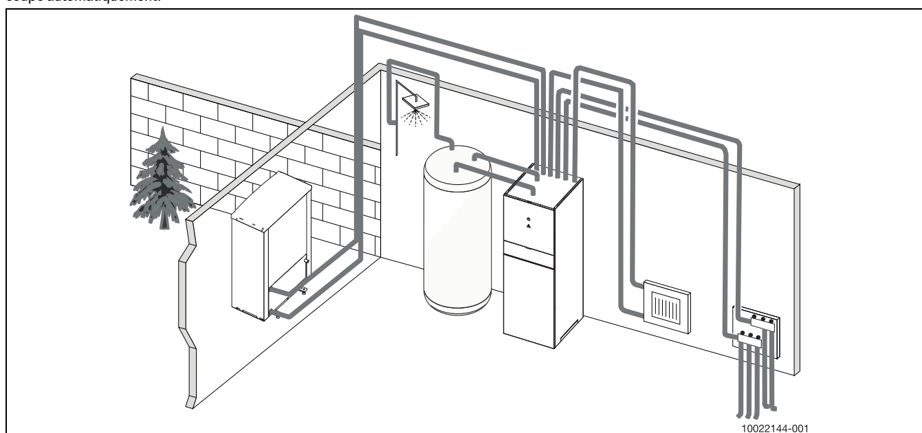
Fig. 3 Pompe à chaleur Compress 7001i AW, unité intérieure AWMB avec ballon tampon intégré et chauffage d'appoint électrique, ballon d'eau chaude sanitaire externe
