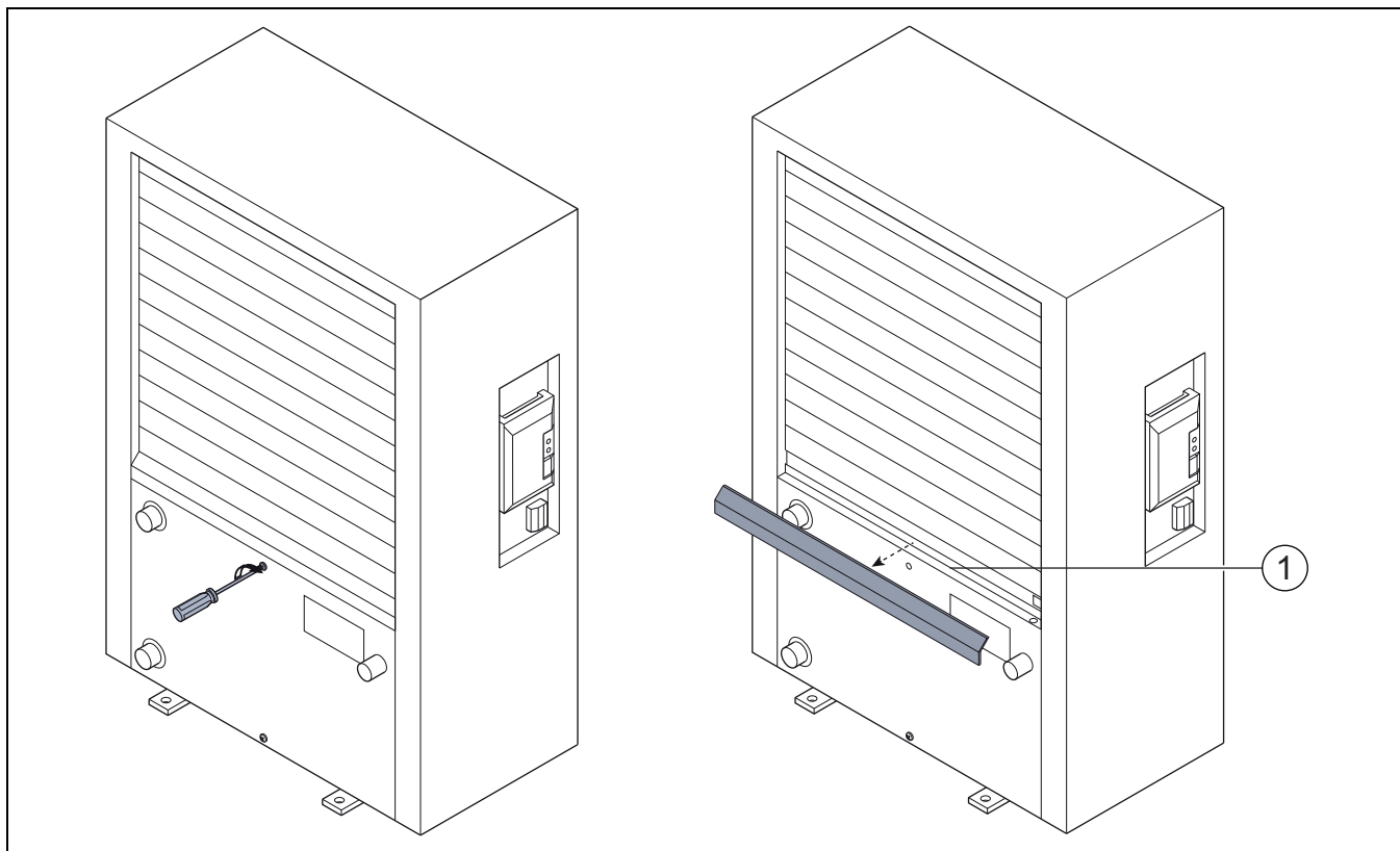
Fig. 9 Réservoir à condensats de la pompe à chaleur
