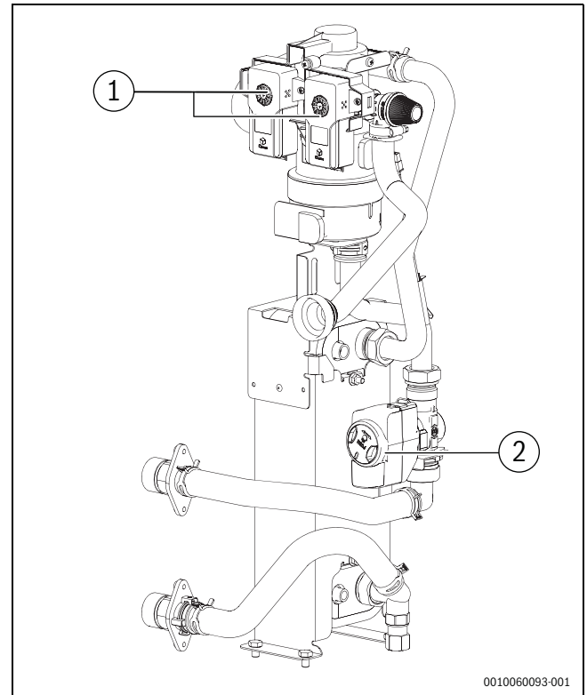
Bild 41 Propan-Sicherheitsset
