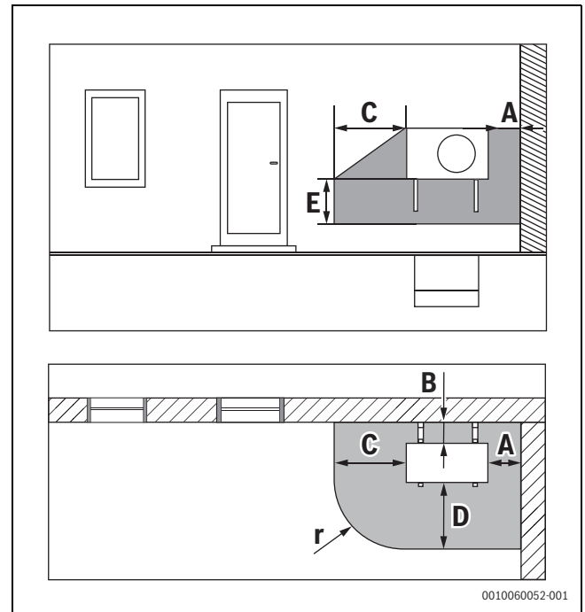
Bild 12 Schutzbereich bei wandhängender Wärmepumpe
