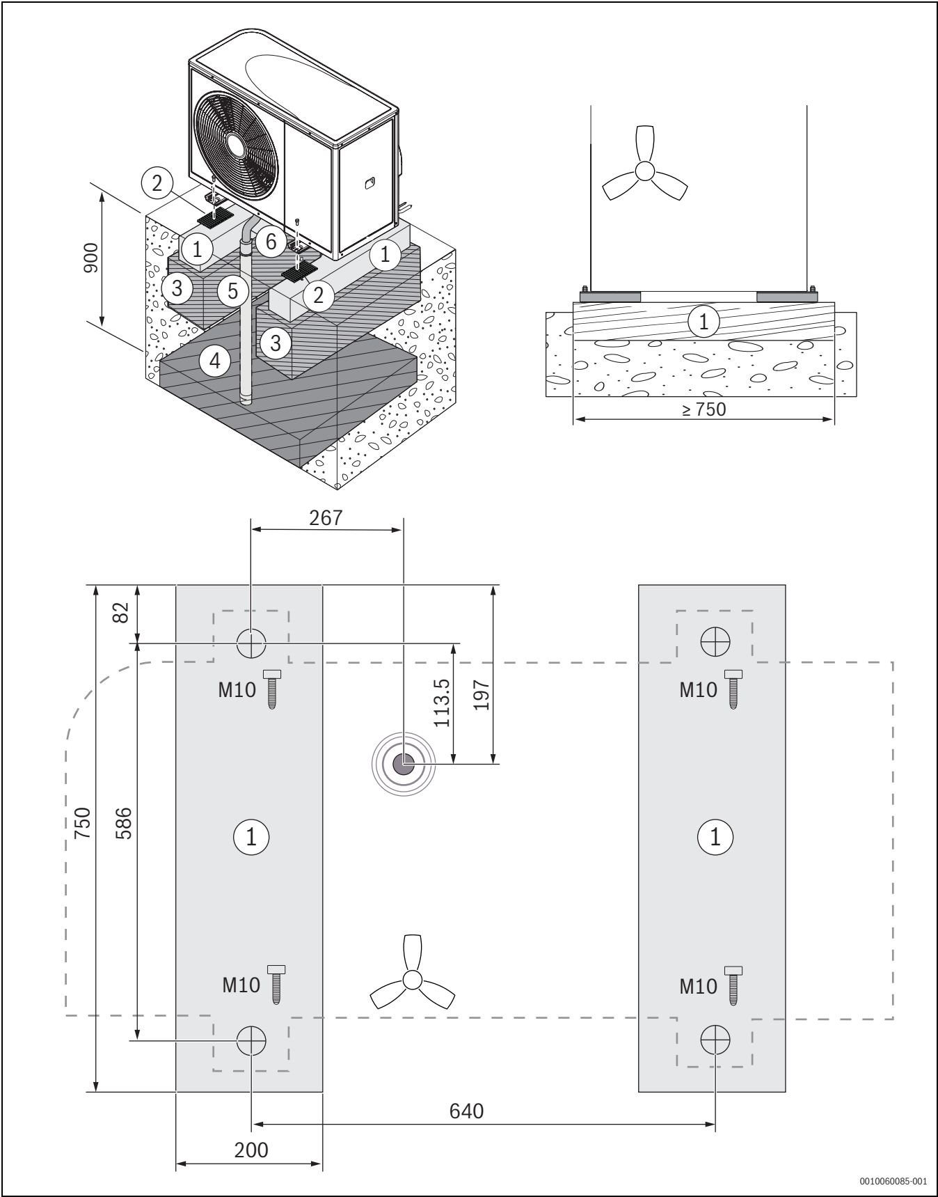
Bild 27 Fundamentplan, Alternative 1
