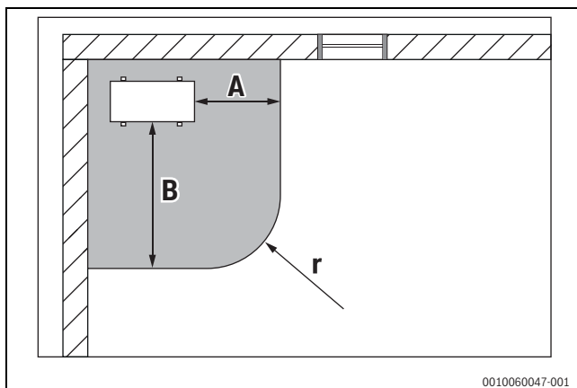
Bild 11 Schutzbereich bei bodenstehender Aufstellung in einer Ecke, Draufsicht
