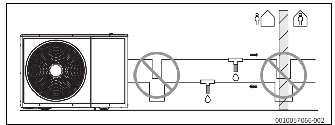
Bild 22 Installation des Frostschutzventils
