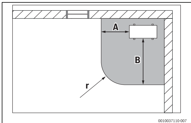
Bild 10 Schutzbereich bei bodenstehender Aufstellung in einer Ecke, Draufsicht
