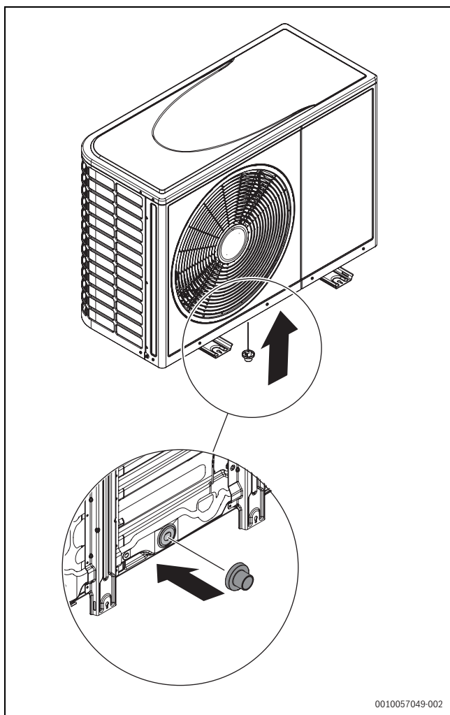
Bild 25 Installation des Abflusstutzens
