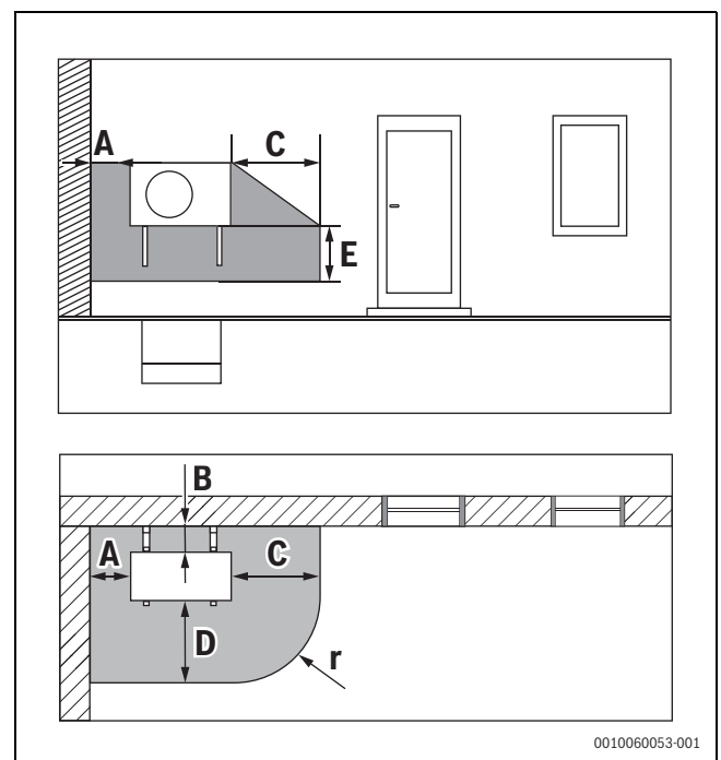
Bild 13 Schutzbereich bei wandhängender Wärmepumpe
