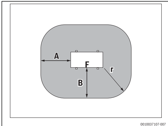
Bild 9 Schutzbereich bei Bodenmontage auf Grundstück oder Dach, Draufsicht
