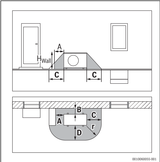
Bild 14 Schutzbereich bei bodenstehender Wärmepumpe an der Wand mit seitlicher Barriere
