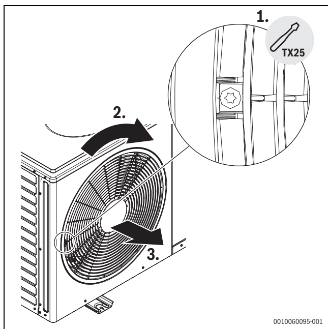
Bild 37 Anleitung für die Demontage der Ventilatorblende
