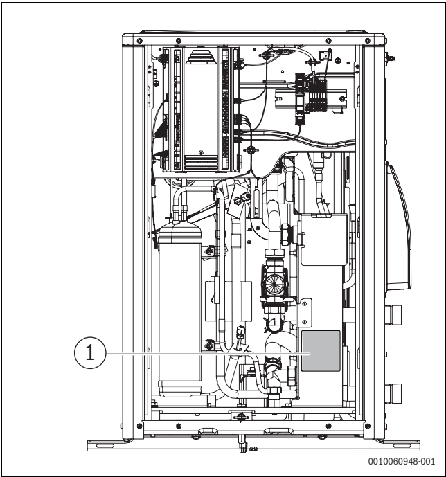
Fig. 5 Emplacement de l'étiquette de la plaque signalétique sur le support PHE
