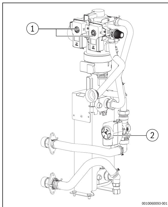
Fig. 41 Kit de sécurité propane
