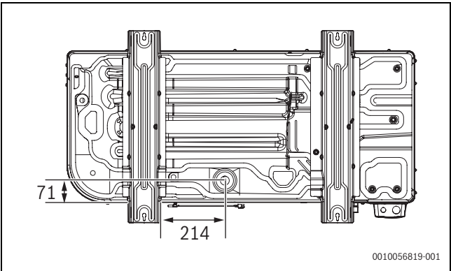
Fig. 7 Dimensions de la pompe à chaleur, vue inférieure
