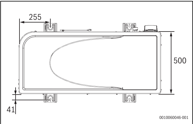
Fig. 6 Dimensions de la pompe à chaleur, vue supérieure
