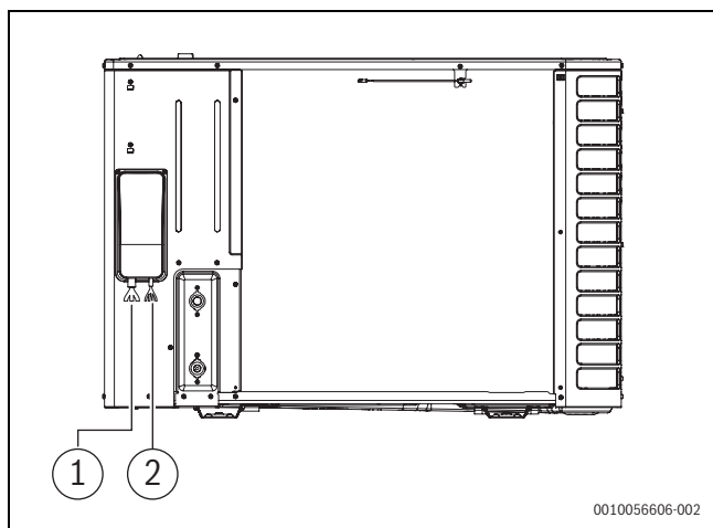
Fig. 33 Presse-étoupes de câbles
