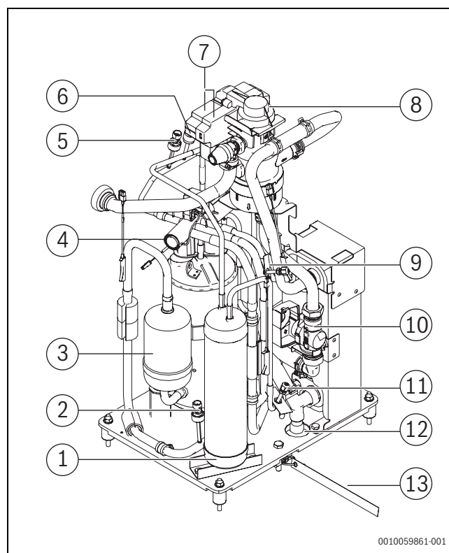
Fig. 2 Vue d'ensemble du circuit de réfrigération
