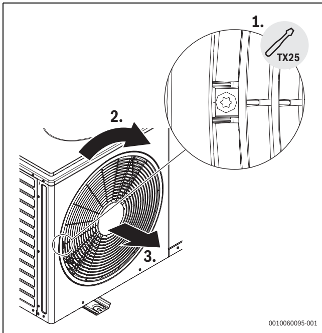
Fig. 37 Instructions relatives au retrait du cadre du ventilateur
