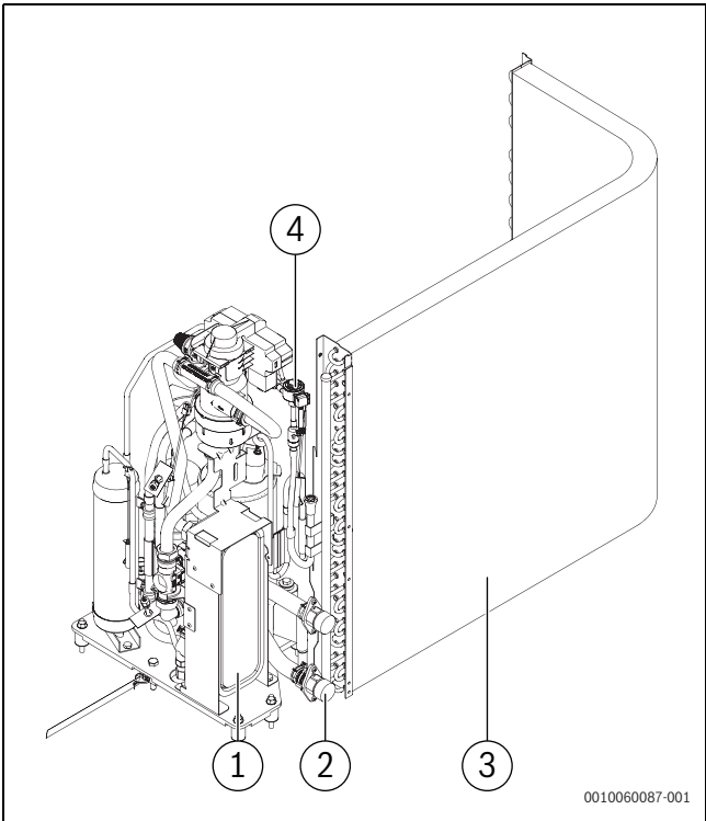
Fig. 3 Vue arrière de la vue d'ensemble du produit
