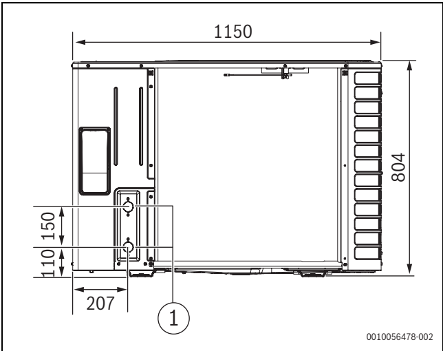
Fig. 4 Dimensions et raccordements hydrauliques de la pompe à chaleur, vue arrière
