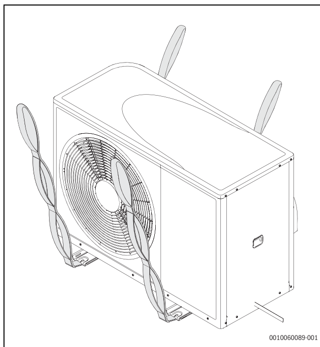
Fig. 17 Utilisation des sangles fournies pour transporter la pompe à chaleur sans son emballage
