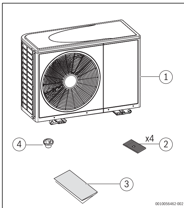
Fig. 1 Composants de l'appareil et de la boîte d'accessoires
