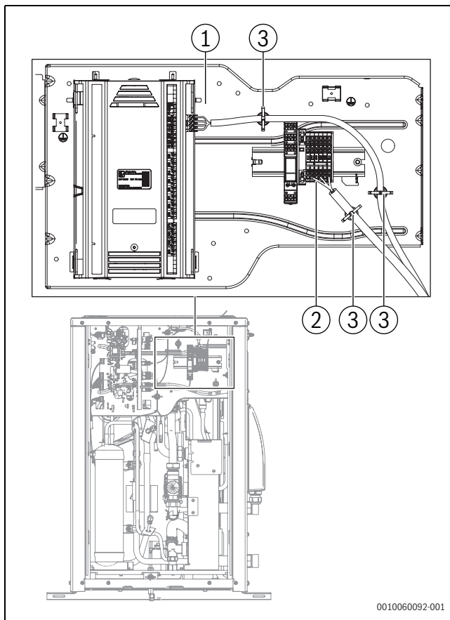
Fig. 36 Bornes de raccordement au niveau de la zone de raccordement de l'installation
