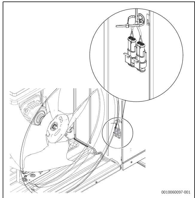
Fig. 39 Élément chauffant du bac de récupération et raccordement du câble de chauffage
