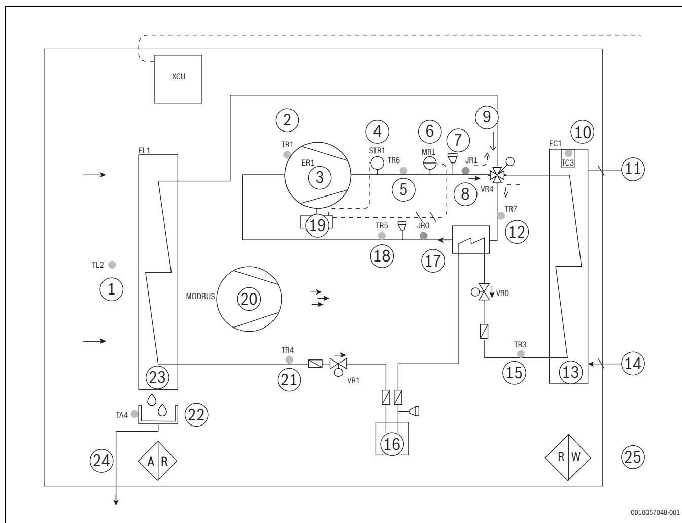
Bild 39 Kältekreis
