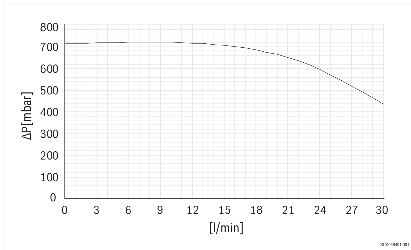
Bild 28 Leistungsdiagramm für die Heizkreispumpe in einem Heizkreis mit konstantem Druck
