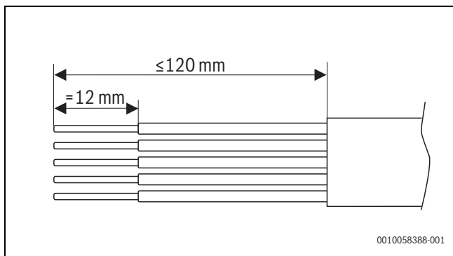
Fig. 45 Spellamento del cavo di alimentazione principale
