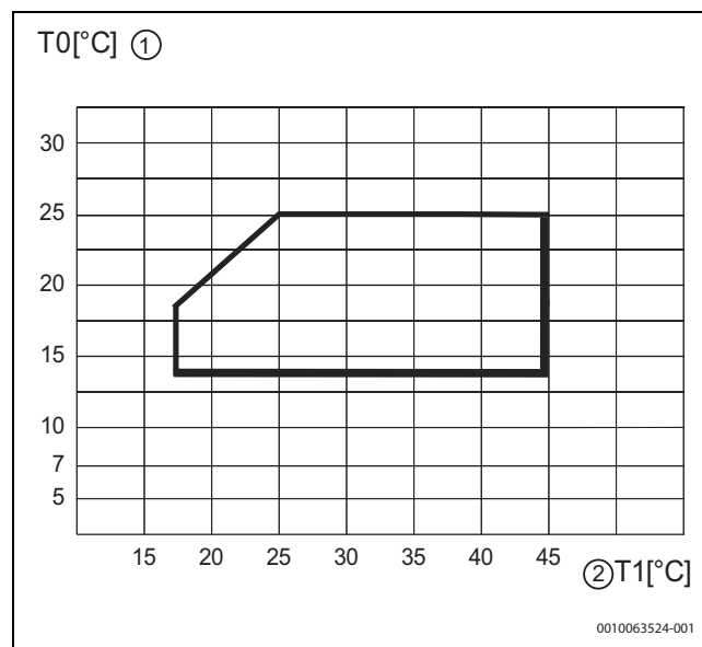
Fig. 25 Pompe à chaleur en mode refroidissement
