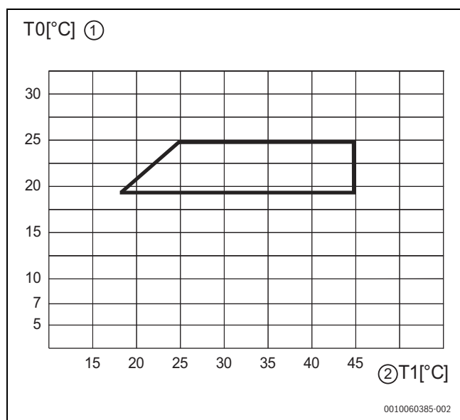
Bild 34 Wärmepumpe im Kühlbetrieb
