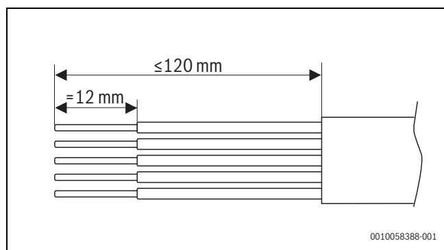
Fig. 42 Spellamento del cavo di alimentazione principale
