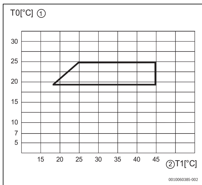
Fig. 21 Pompe à chaleur en mode refroidissement
