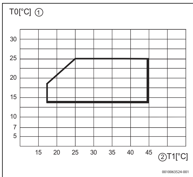
Bild 38 Wärmepumpe im Kühlbetrieb
