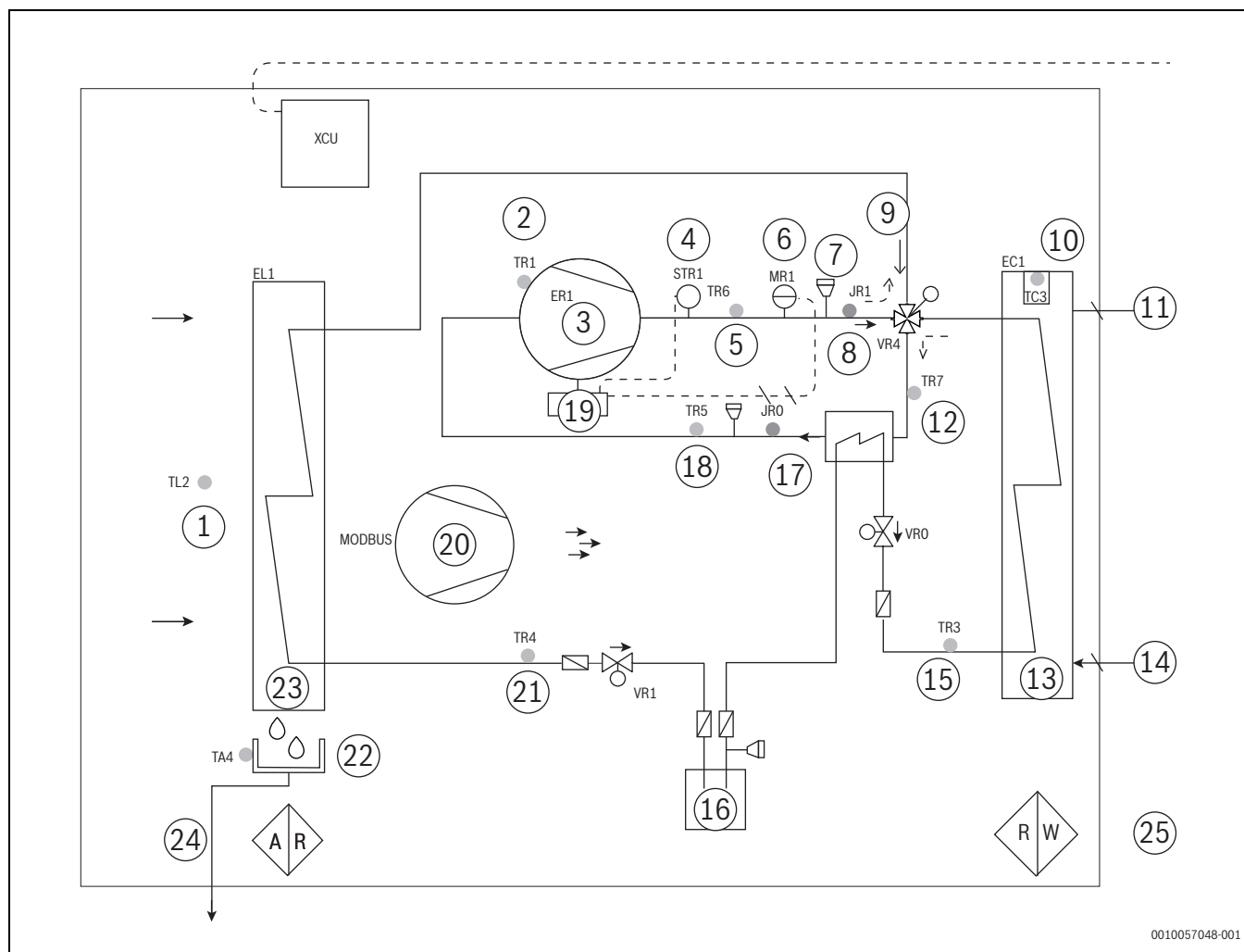
Fig. 52 Circuito frigorifero
