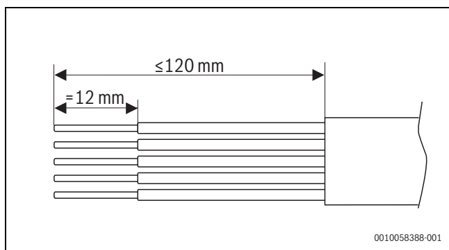
Fig. 19 Raccordement à l'alimentation secteur avec dénudage des fils
