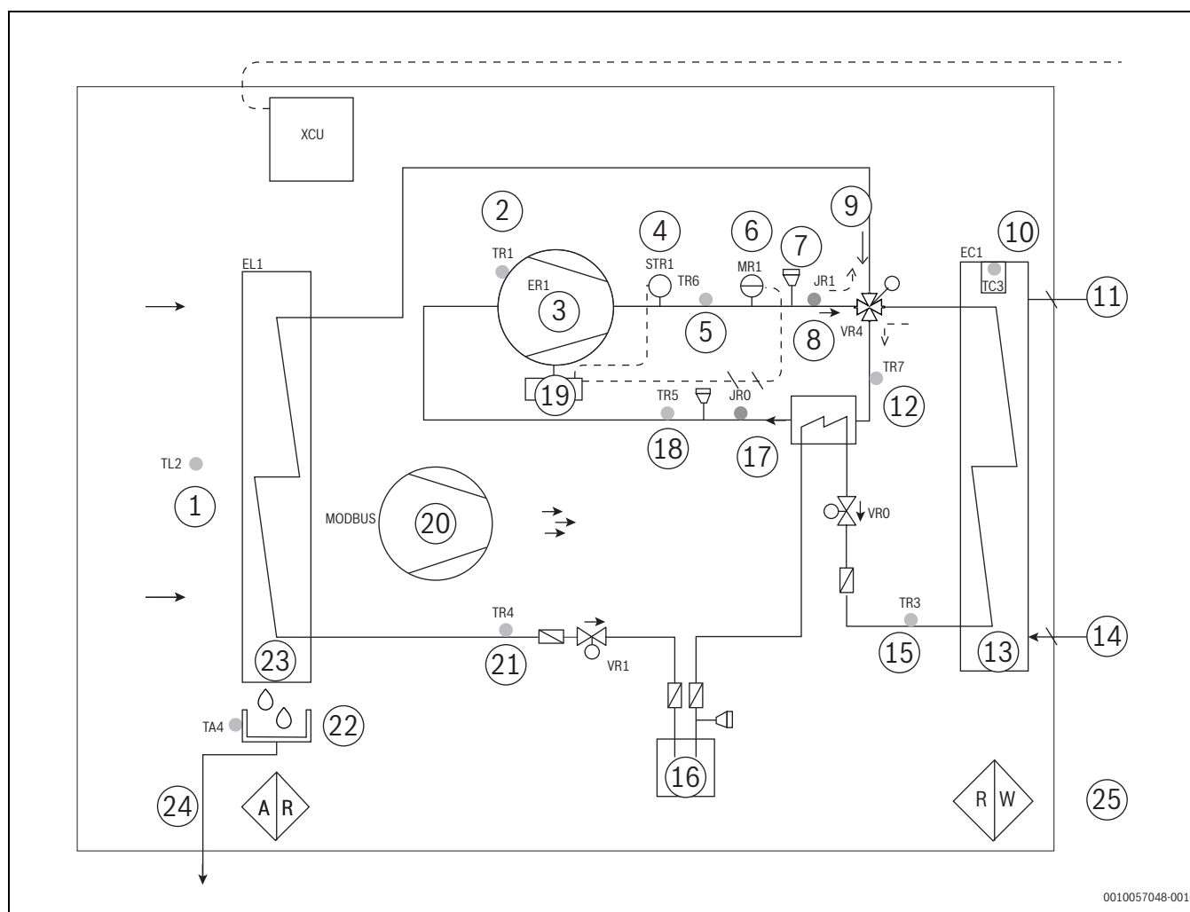
Fig. 26 Circuit frigorifique
