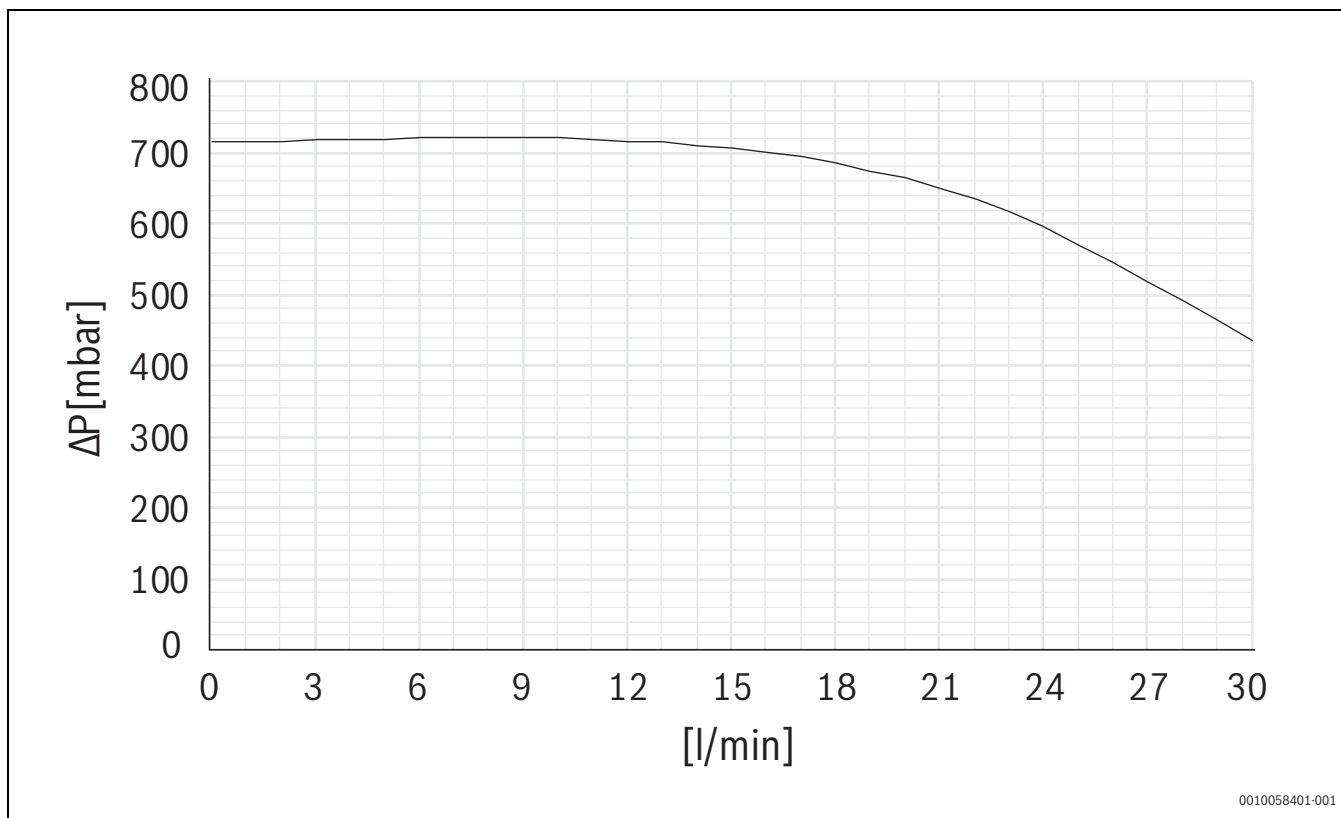
Fig. 15 Graphique de performance de la pompe du circuit de chauffage dans un circuit de chauffage à pression constante
