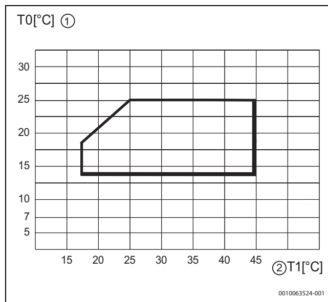
Fig. 51 Pompa di calore in modalità raffrescamento
