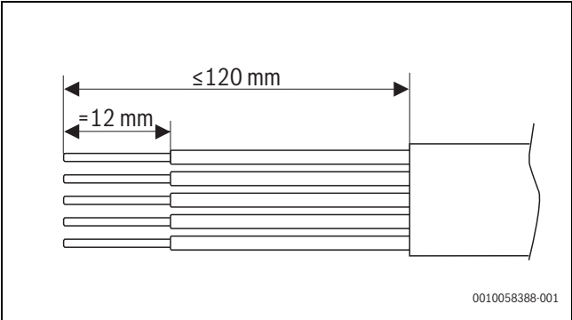
Fig. 16 Dénudage des fils pour le raccordement de l'alimentation secteur
