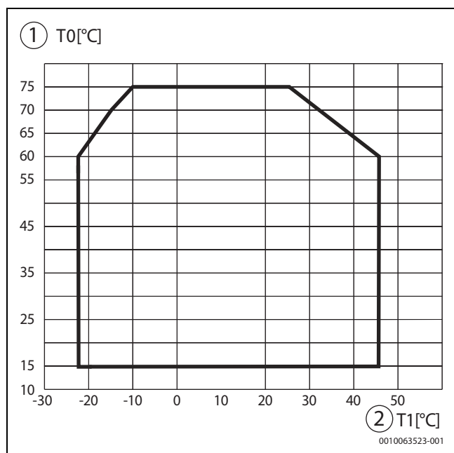
Fig. 50 Pompa di calore in modalità riscaldamento senza riscaldatore ausiliario
