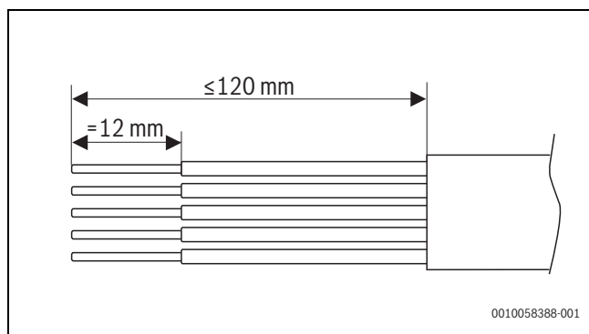
Bild 29 Abisolieren der Adern für den Netzanschluss
