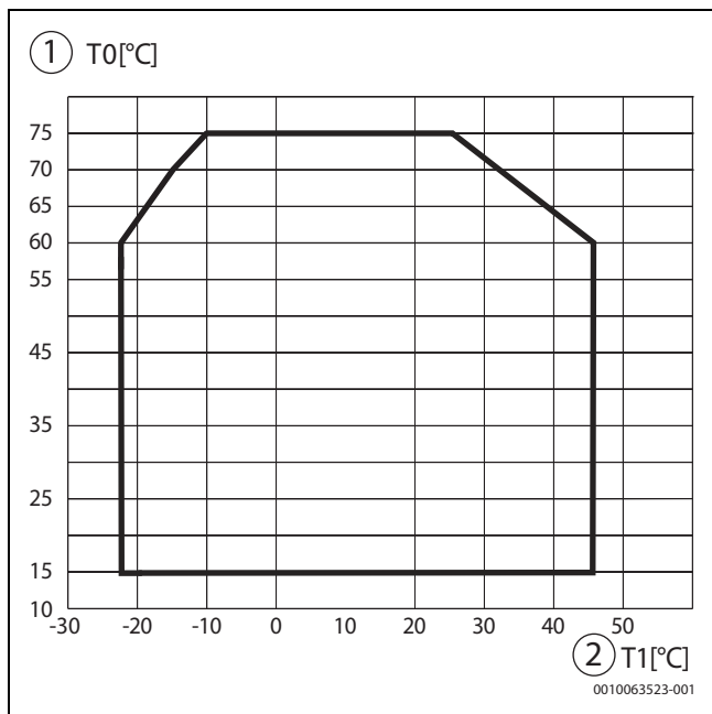
Bild 37 Wärmepumpe im Heizbetrieb ohne Zuheizung
