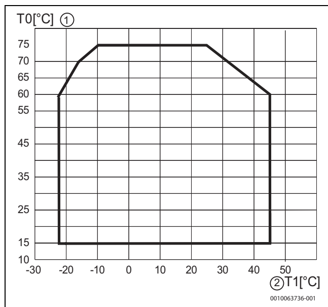
Fig. 20 Pompe à chaleur en mode chauffage sans chauffage d'appoint électrique
