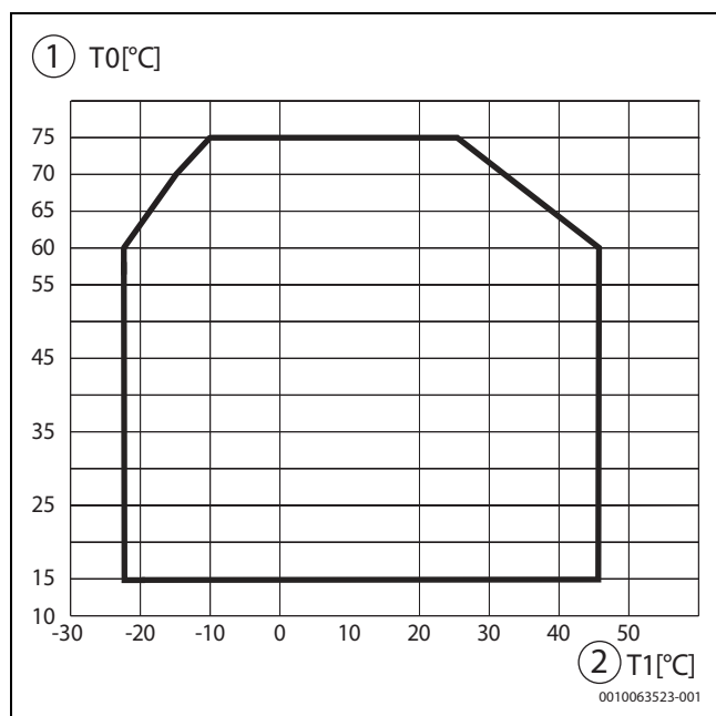
Fig. 24 Pompe à chaleur en mode chauffage sans appoint
