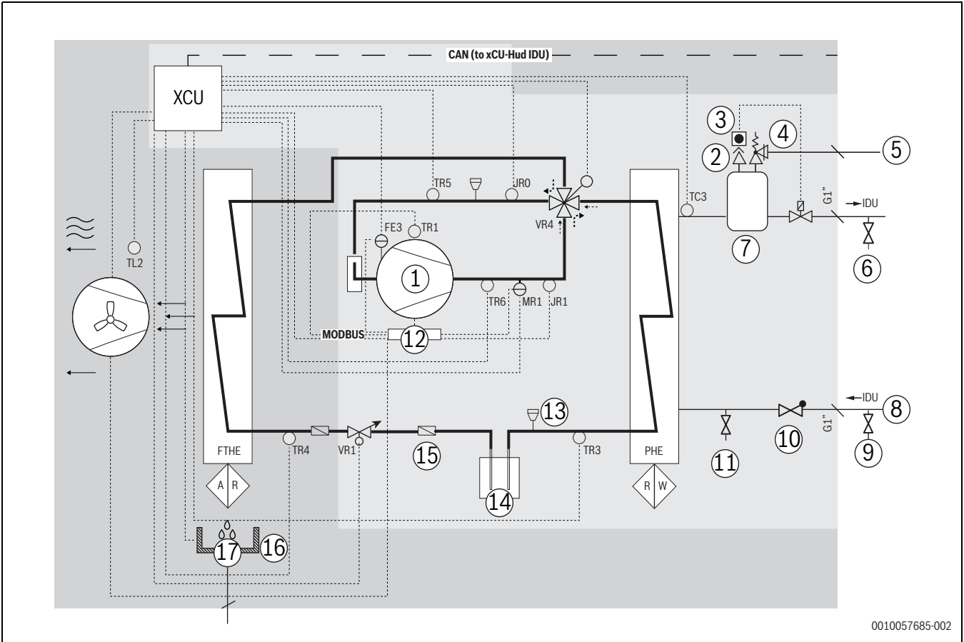
Bild 9 Kältekreis
