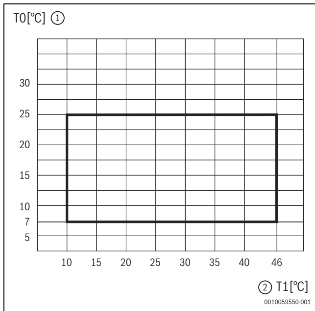
Fig. 38 Pompa di calore in modo raffreddamento
