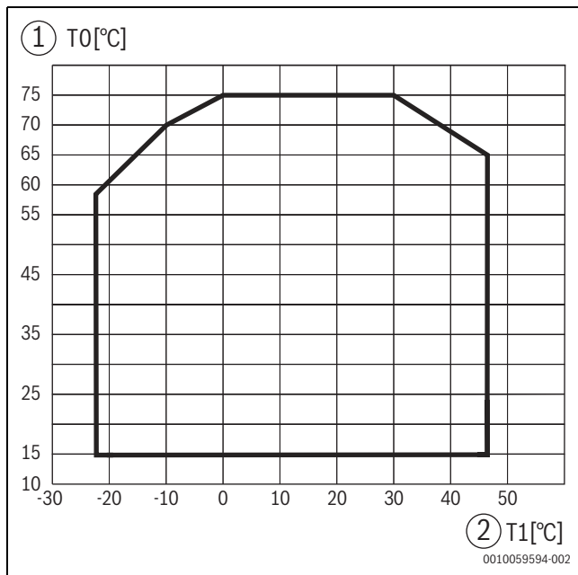
Afb. 52 Warmtepomp in verwarmingsbedrijf zonder bijverwarming.
