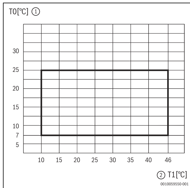
Afb. 68 Warmtepomp in koelbedrijf
