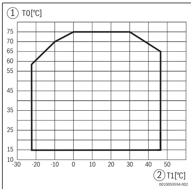
Afb. 67 Warmtepomp in cv-bedrijf zonder bijverwarming
