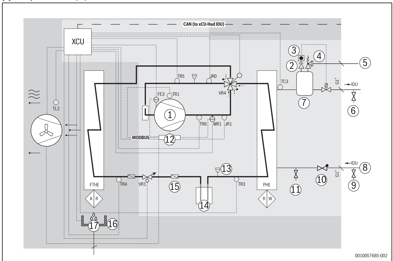
Fig. 38 Pompa di calore in modo raffreddamento
