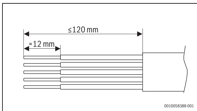
Rys. 79 Usuwanie izolacji z przewodu zasilania sieciowego
