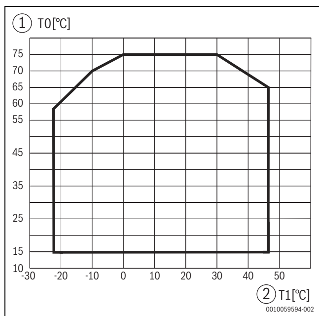
Rys. 82 Pompa ciepła w trybie grzania, bez dogrzewacza
