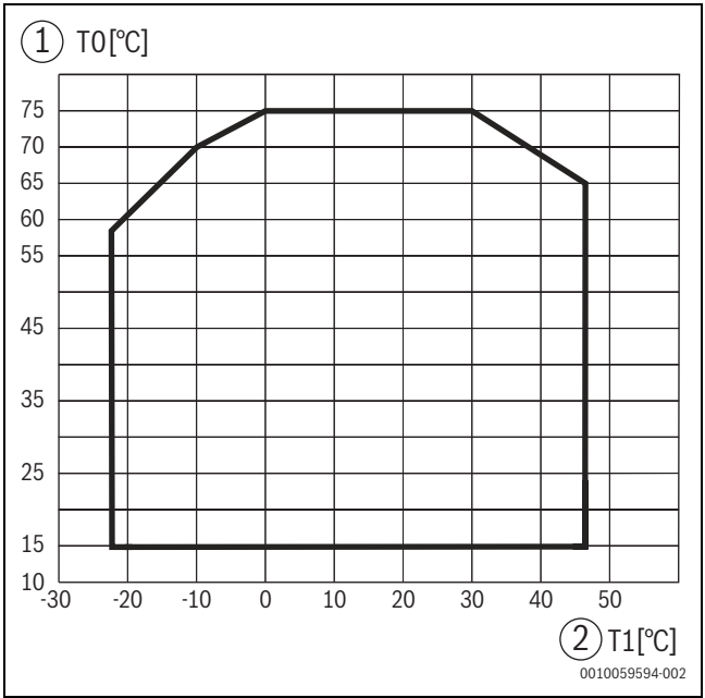
Fig. 37 Pompa di calore in modo riscaldamento senza generatore di calore supplementare
