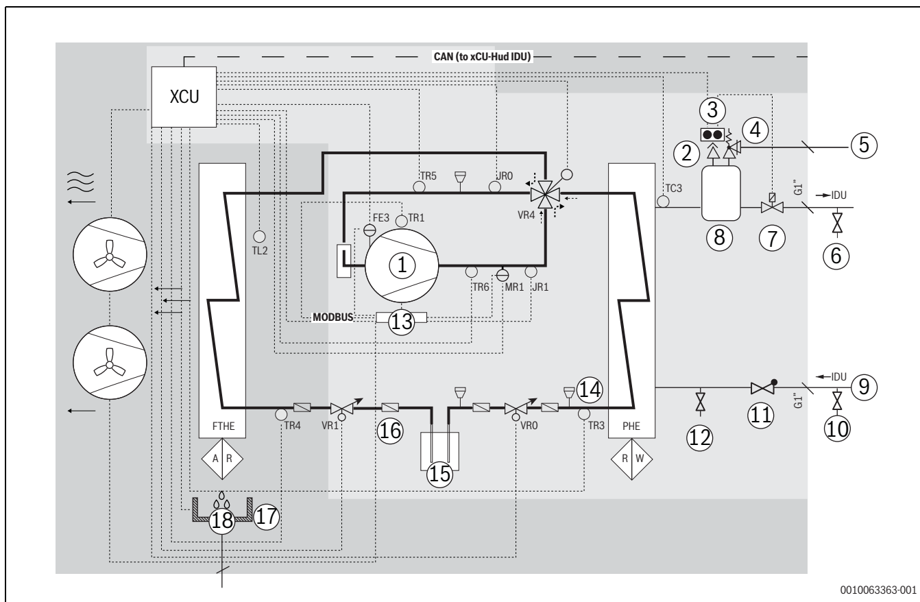
Rys. 88 Obieg czynnika chłodniczego
