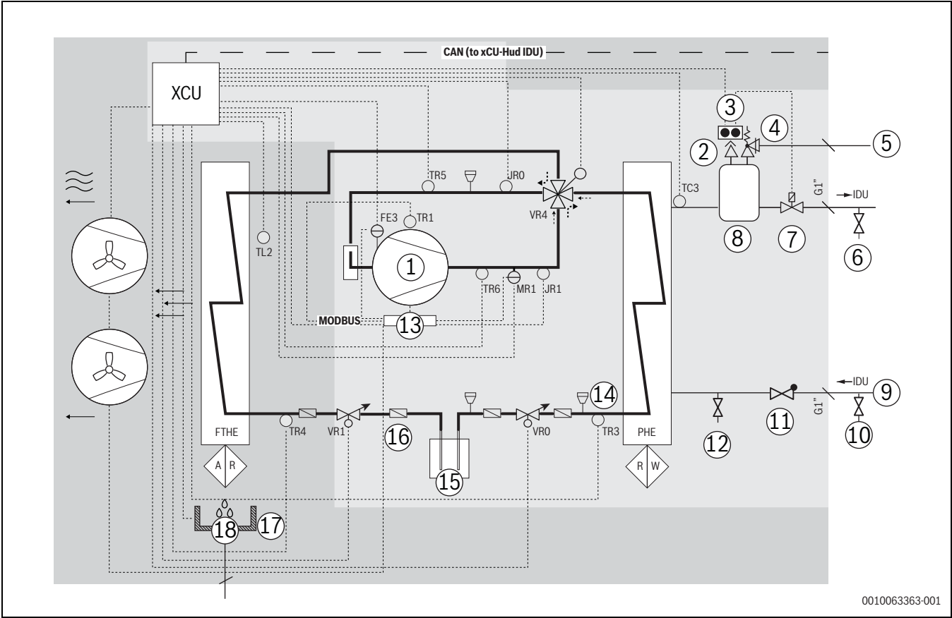
Afb. 73 Koudemiddelcircuit
