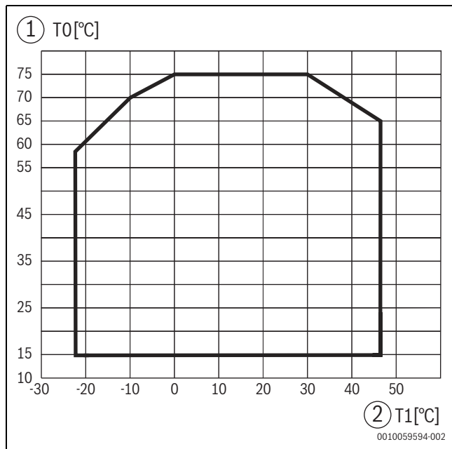
Fig. 22 Pompe à chaleur en mode Chauffage sans appoint électrique
