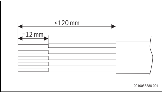
Afb. 49 Aders strippen aansluiting voedingsspanning
