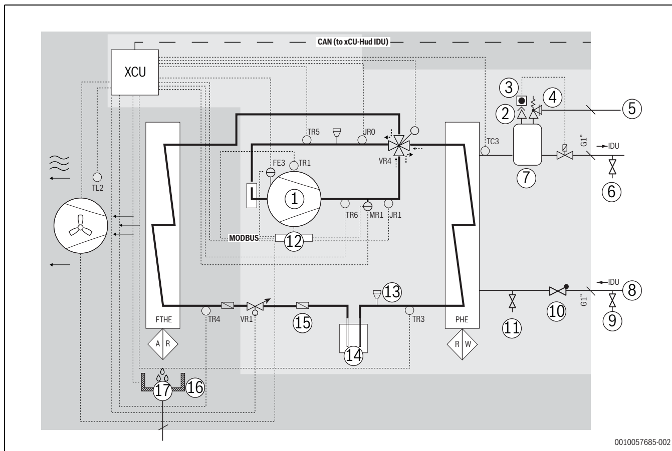
Rys. 84 Obieg czynnika chłodniczego
