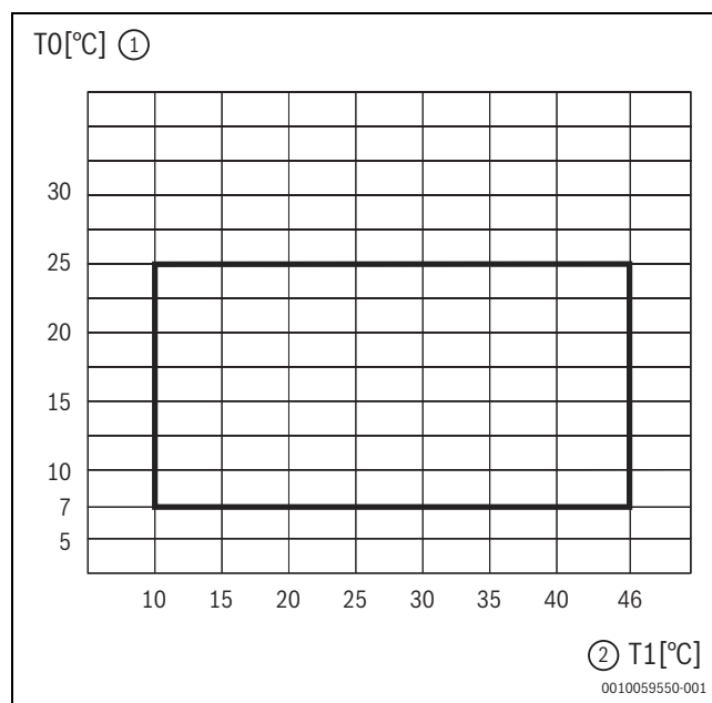
Rys. 83 Pompa ciepła w trybie chłodzenia
