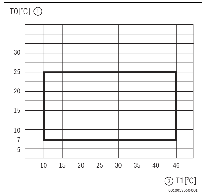
Fig. 23 Pompe à chaleur en mode Refroidissement
