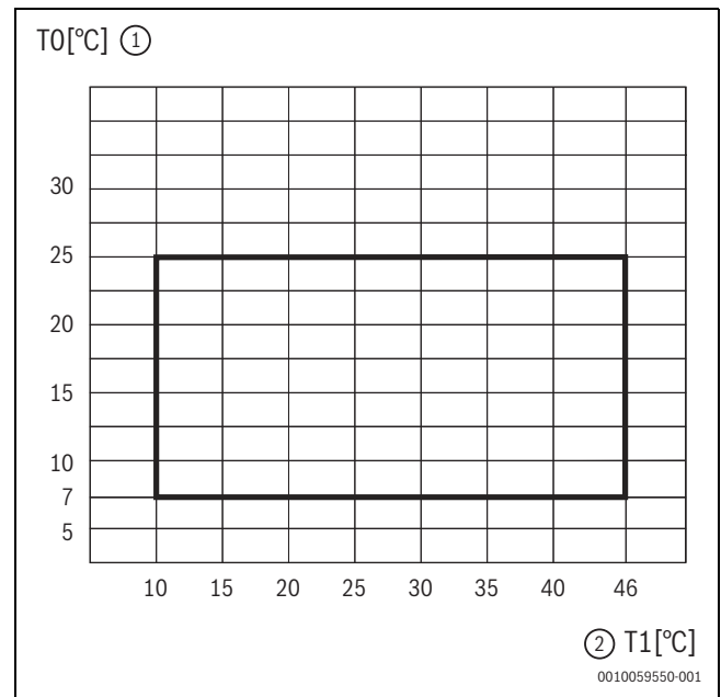
Afb. 53 Warmtepomp in koelmodus
