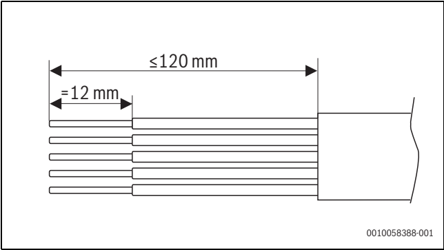
Afb. 64 Striplengte ader voedingsaansluiting
