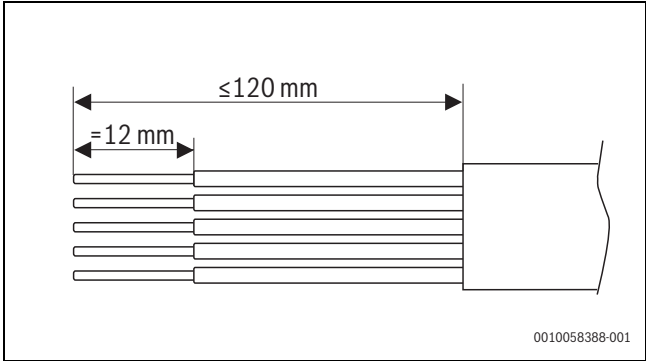
Bild 4 Abisolieren der Adern für den Netzanschluss
