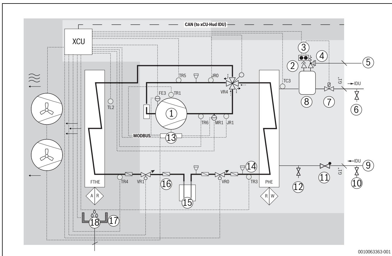
Bild 13 Kältekreis
