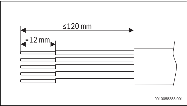
Fig. 34 Spellamento del cavo di alimentazione principale
