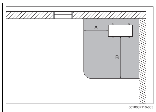
Fig. 3 Zona di sicurezza per installazione a basemento in un angolo
