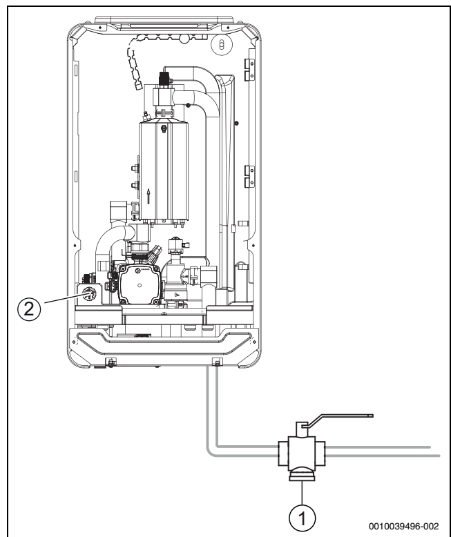
Fig. 13 Unità interna Compress 5800/6800i 12 E
