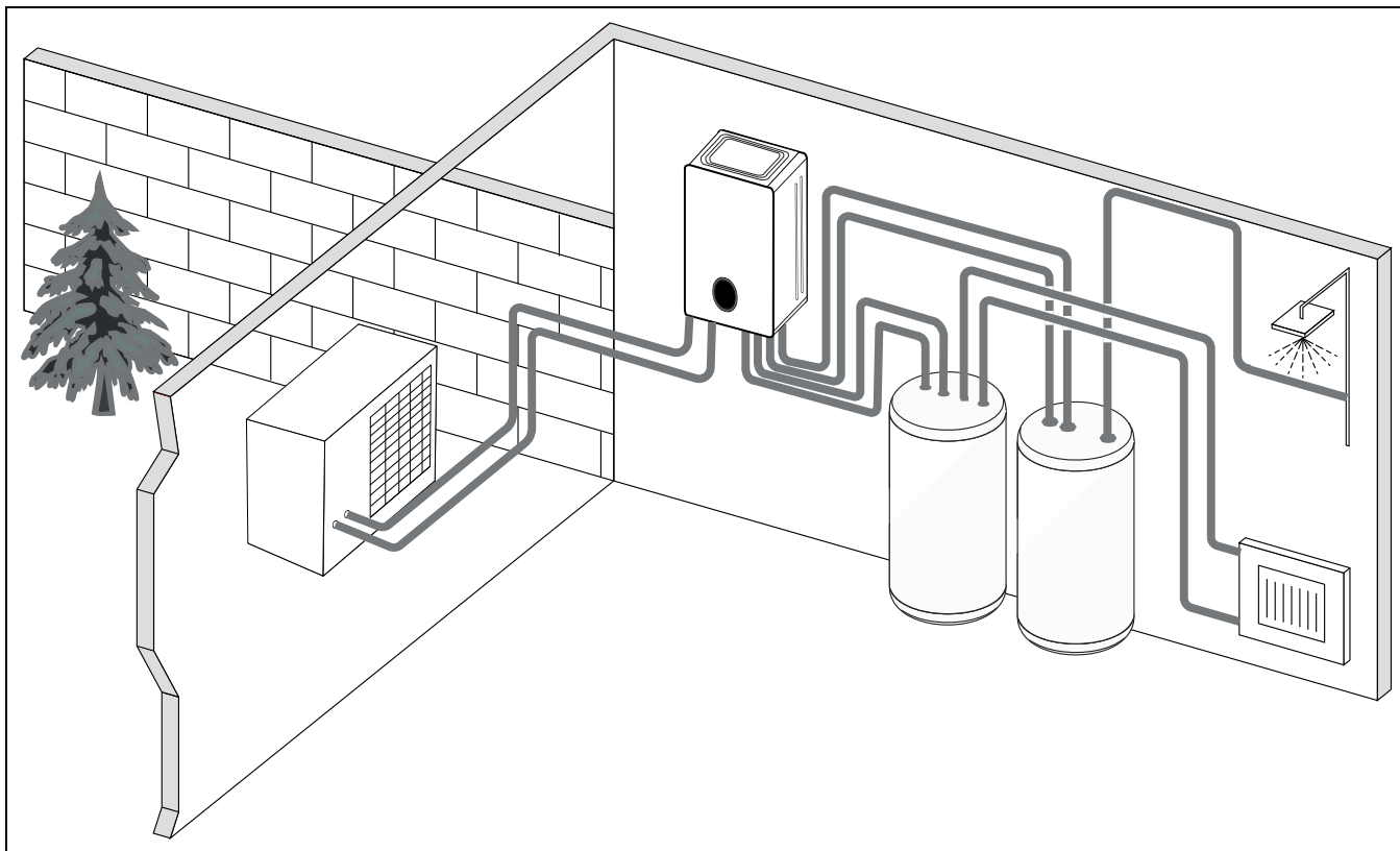
Fig. 7 Pompa di calore AW OR, unità interna Compress 5800/6800i 12 E con resistenza elettrica integrata e bollitore di acqua calda sanitaria esterno
