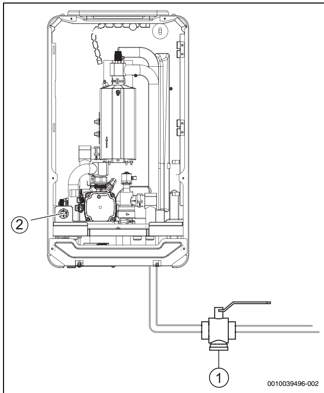
Fig. 13 Unité intérieure Compress 5800/6800i 12 E
